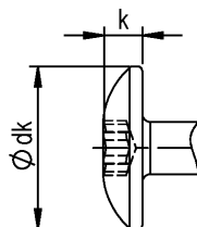
Flachrundkopf
