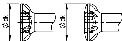
Kleiner (Linsensenk-) Kopf
