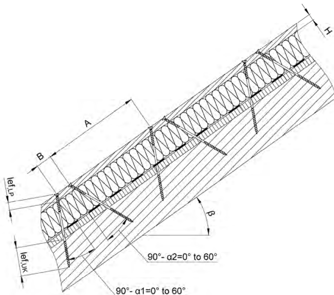
Abbildung A.4.4 Befestigung der Aufdach-Dämmung auf Sparren – Prinzipdarstellung mit wechselnder Neigung angeordneter Schrauben und durchlaufende Konterlatte beansprucht aus konstanter Linienlast auf die Dachfläche q_{\perp} und Einzellasten aus den zugbeanspruchten Schrauben F_{Zs}
